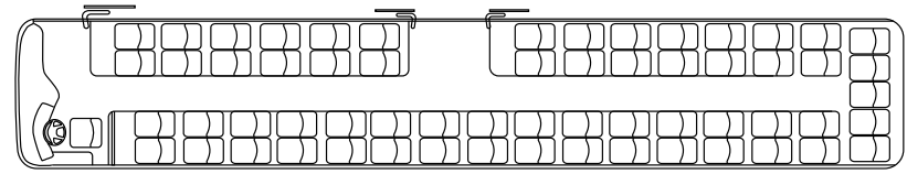
Penkkikaavio: 61+0+1 (WC) / esimerkki
