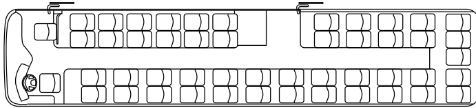
Penkkikaavio: 47+1+1 (WC) / esimerkki
